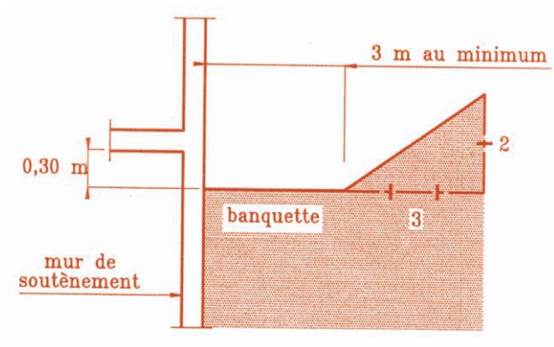
Figure 6-2 : Banquette derrière le mur de soutènement
