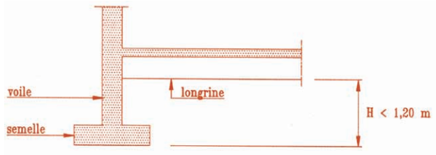
Figure 6-1 : Fondation du mur de soutènement
