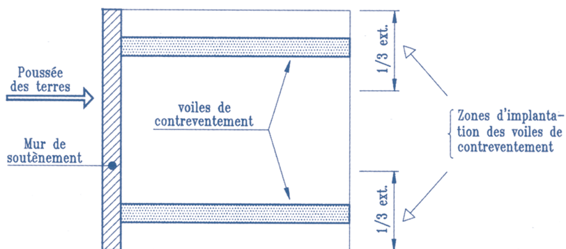
Figure 6-3 : Contreventement des murs de soutènement
